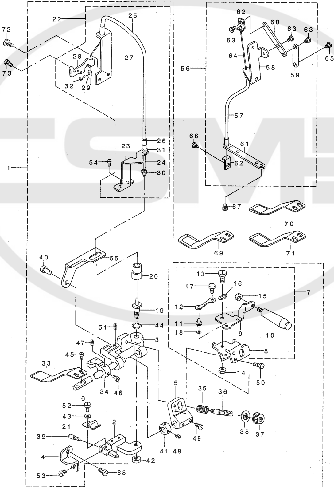
SWING TYPE KNEE DIFFERENTIAL INTERMITTENT SHIRRING ATTACHMENT(PEDAL TYPE) スイング式膝差動上ひだ取り装置 (ペダル式)
